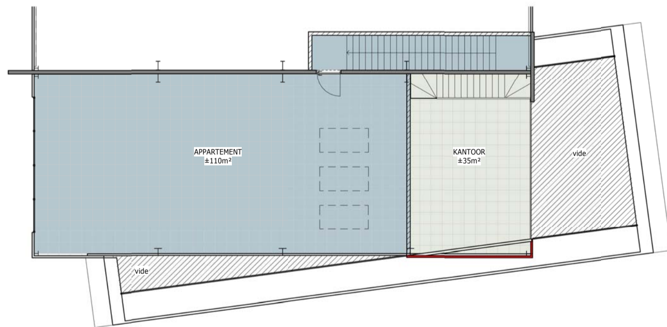
VERDIEPING 1 : 150
