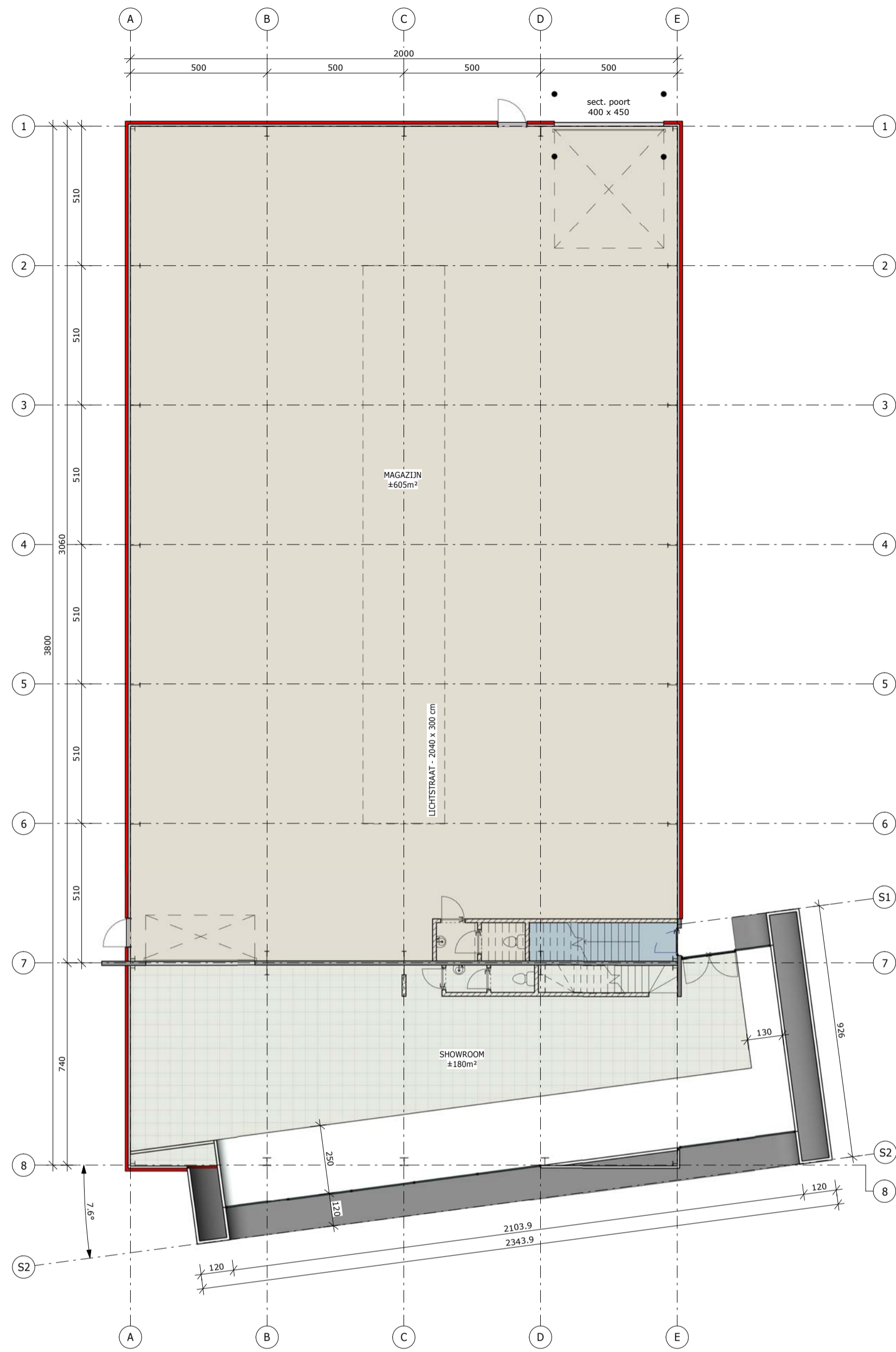
GELIJKVLOERS 1 : 150
