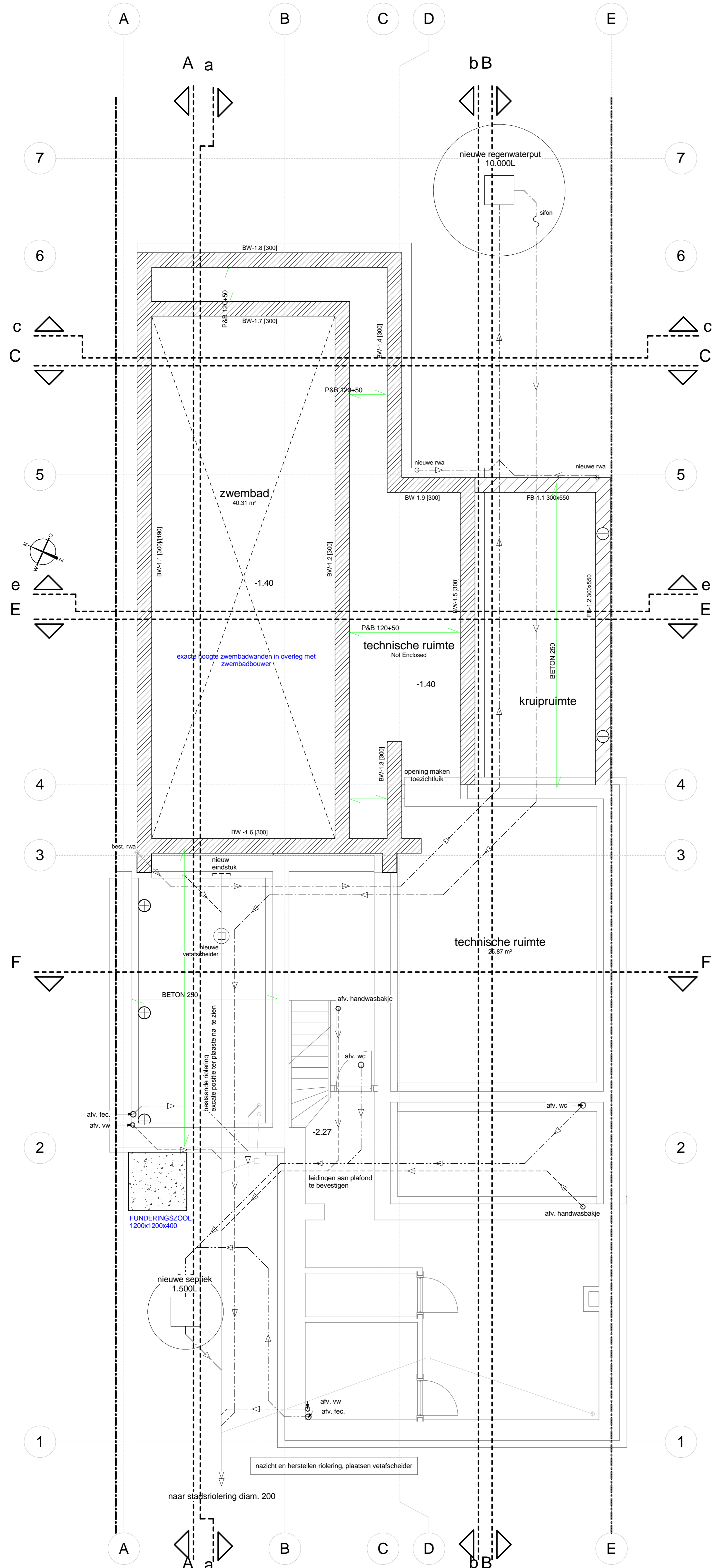
KELDER nieuw 1 : 50
