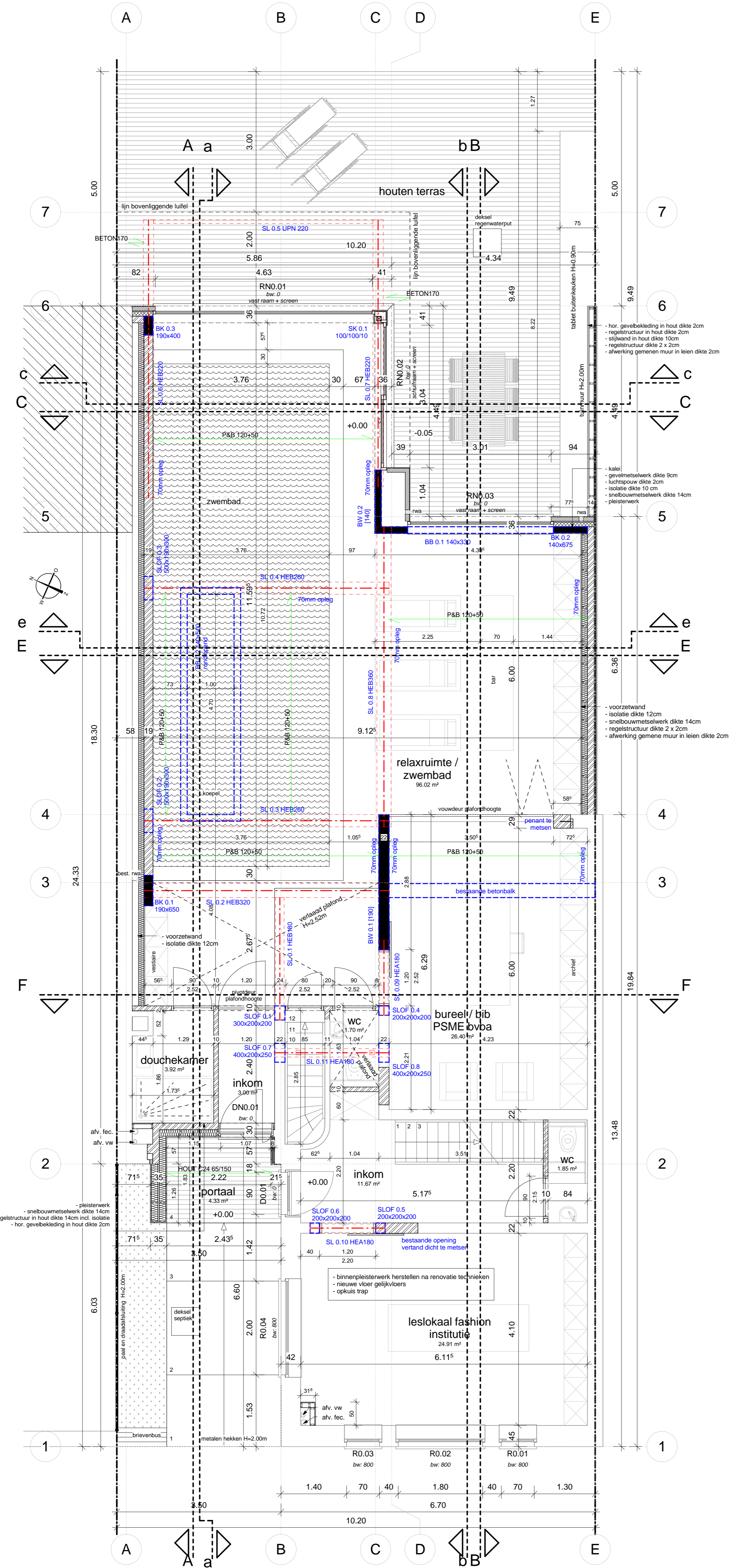
GELIJKVLOERS nieuw 1 : 50
