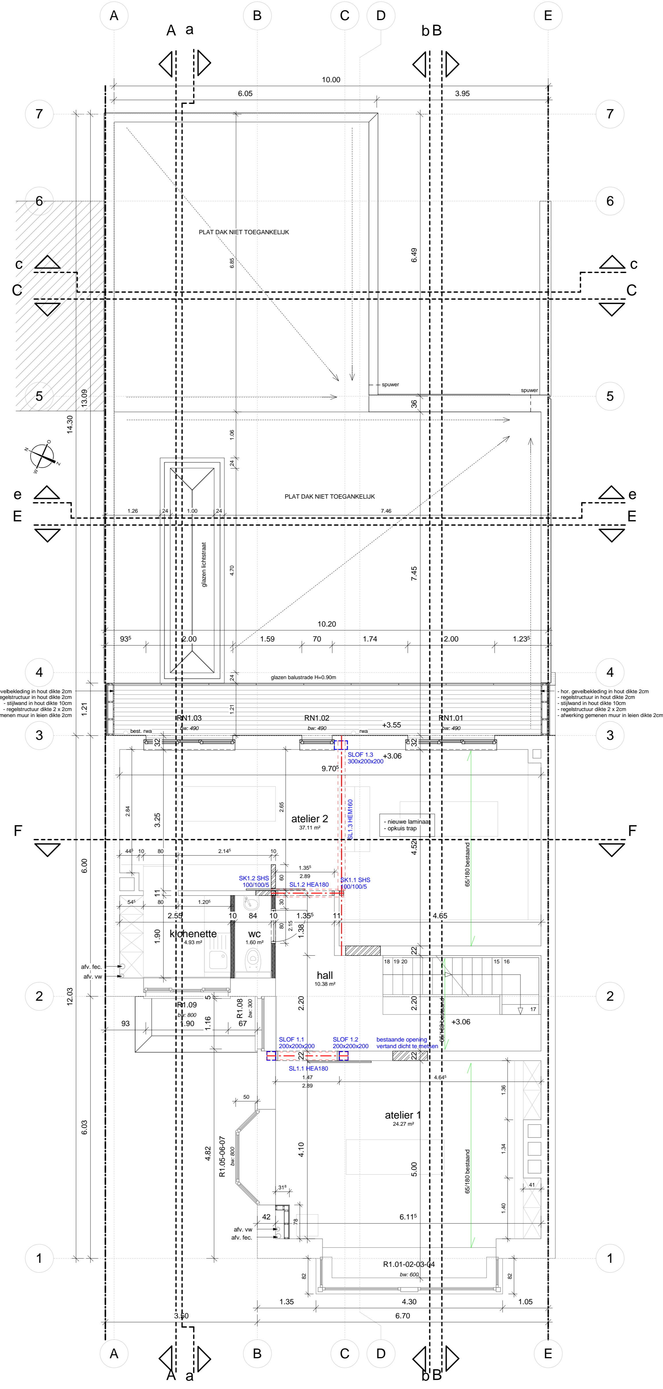
VERDIEPING nieuw 1 : 50
