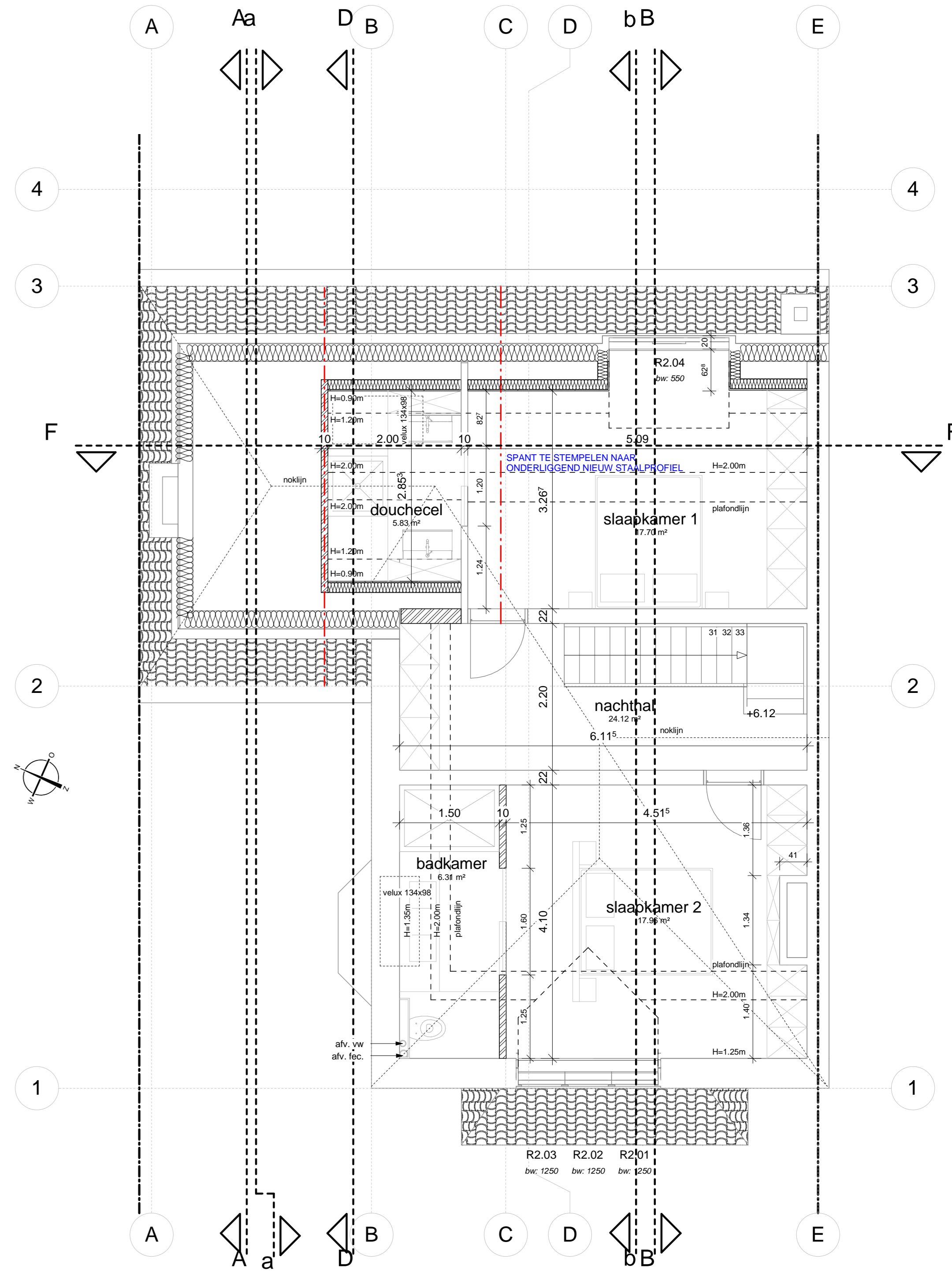
ZOLDER nieuw 1 : 50
