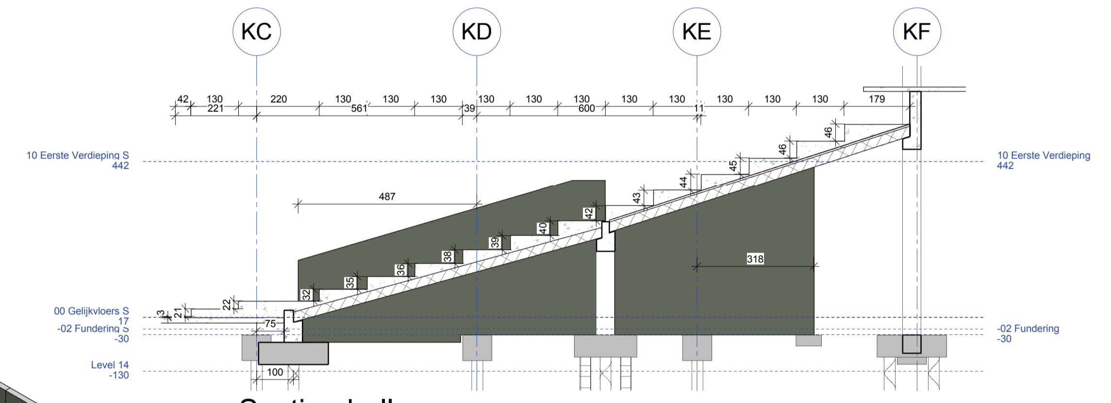
2 Section hall 1 : 100
