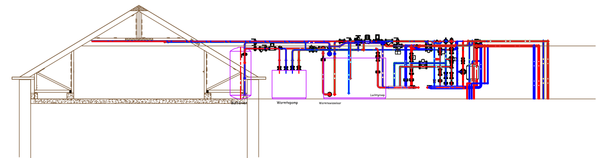
Vooranzicht CV
