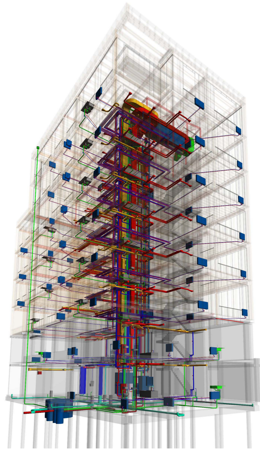
INTEGRATIE TECHNIEKEN
