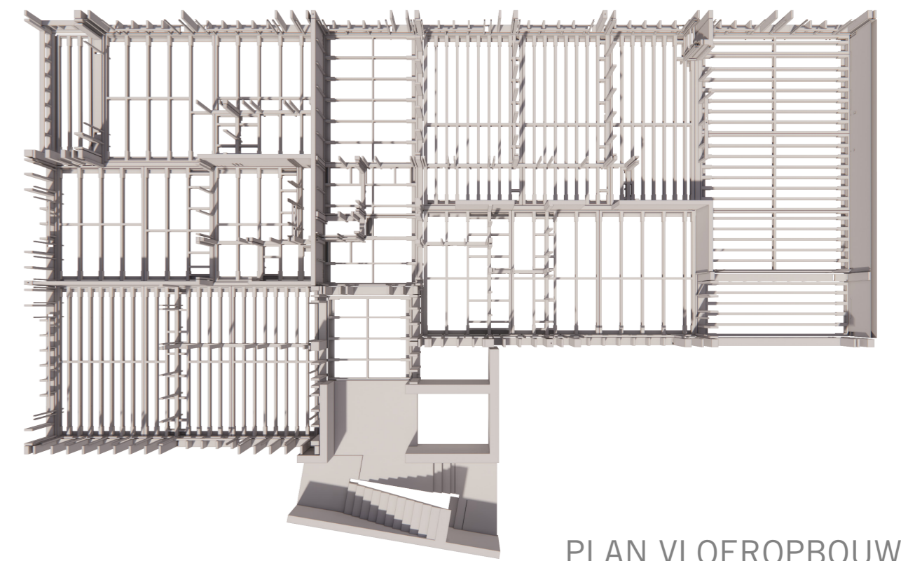
PLAN VLOEROPBOUW
