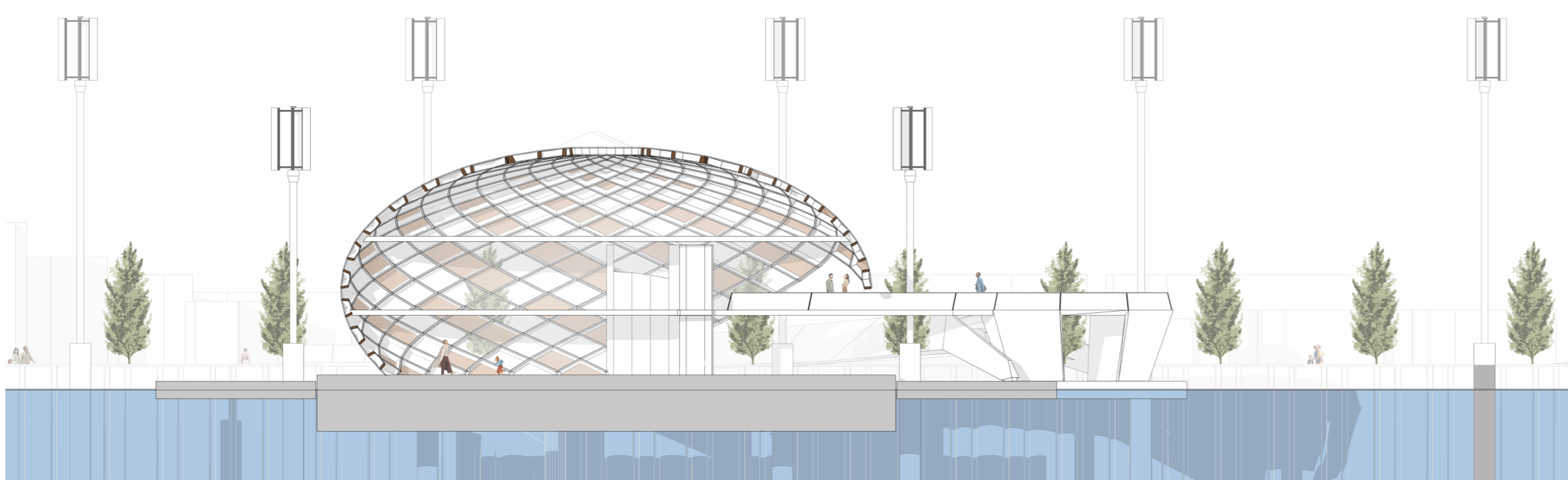
Section A-A'
