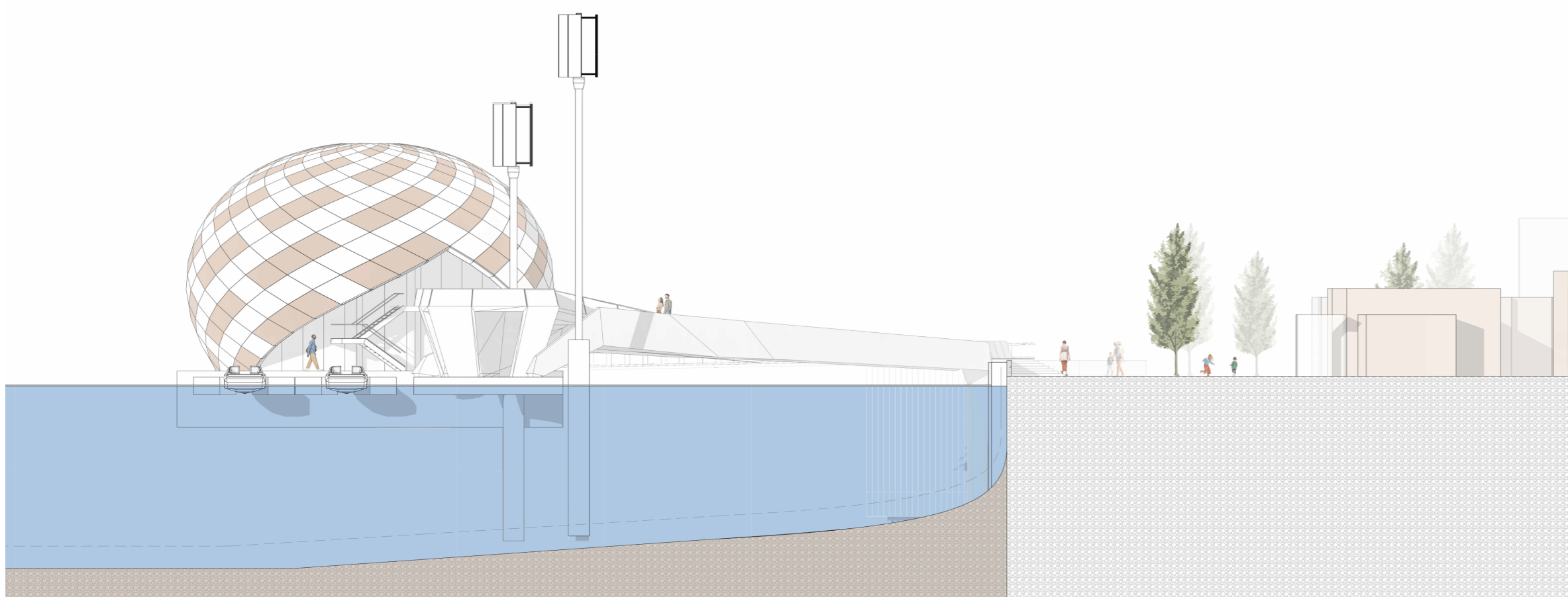
Section A-A'
